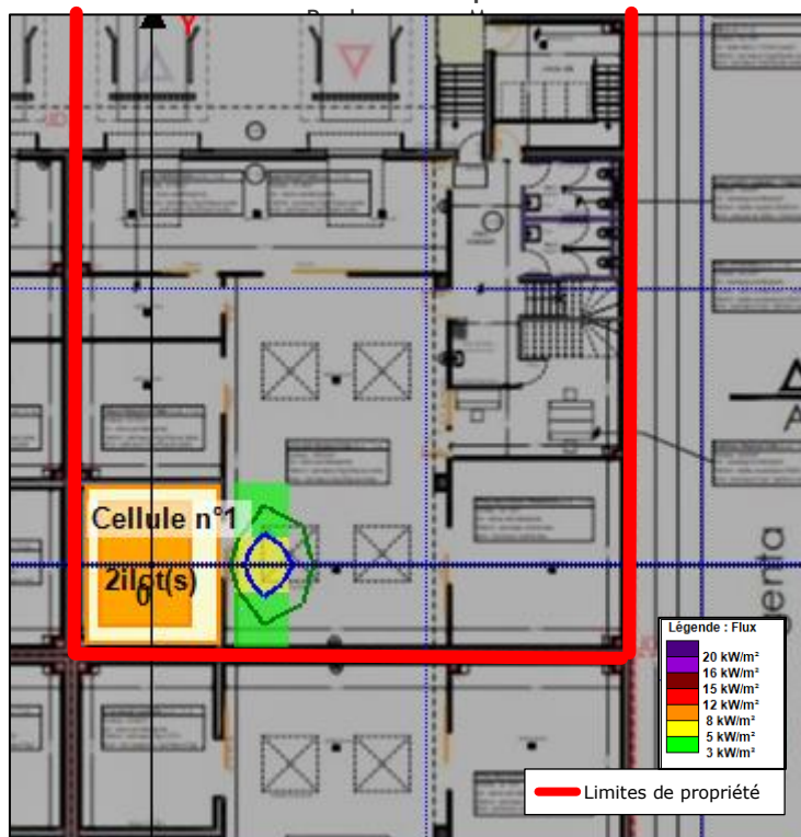
Figure 5. Représentation graphique effets thermiques générés par un incendie sur le stockage des caisses vides
