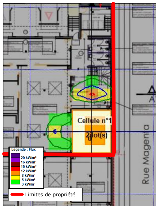
Figure 2. Représentation graphique effets thermiques générés par un incendie sur le stockage frigorifique de matières premières
