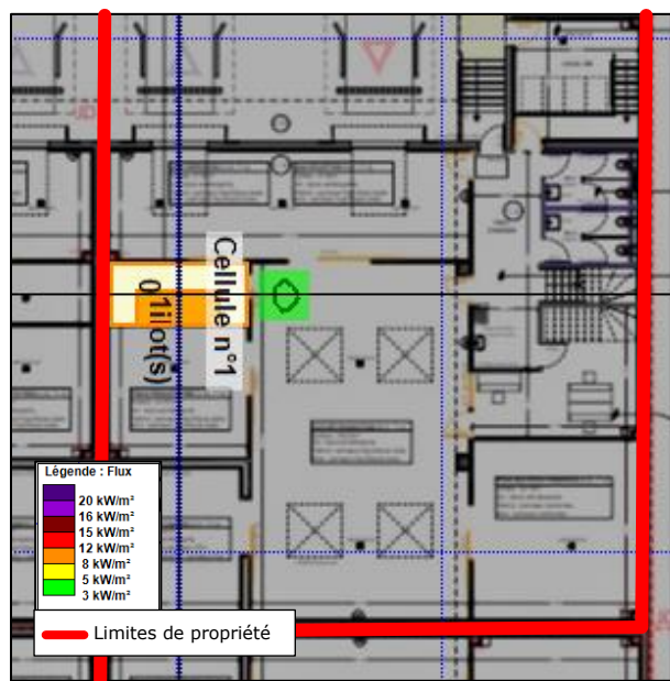
Figure 3. Représentation graphique des effets thermiques générés par un incendie sur le stockage frigorifique des co-produits
