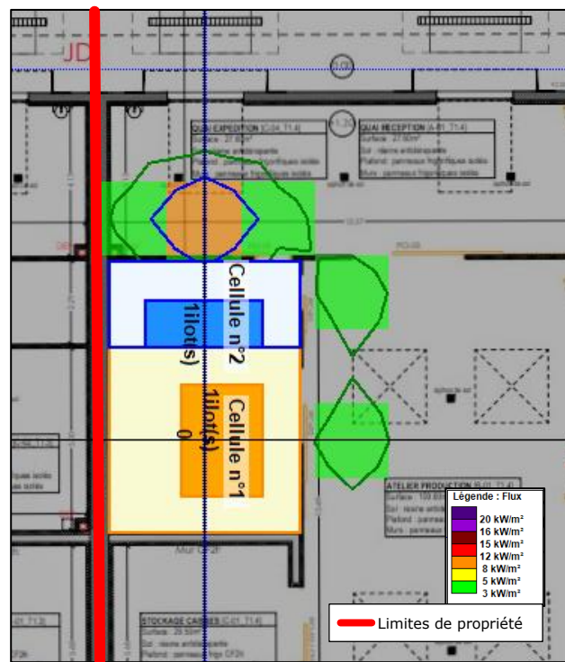
Figure 6. Représentation graphique effets thermiques générés par la propagation
